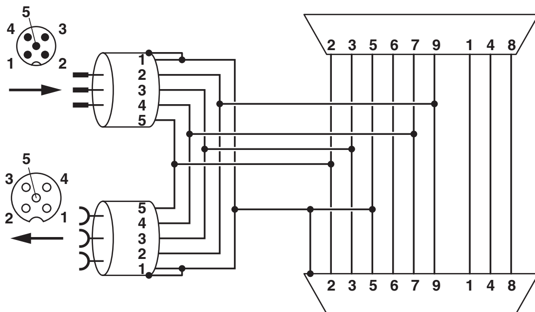
Schema di funzionamento SUBCON-PLUS-CAN/...M12
