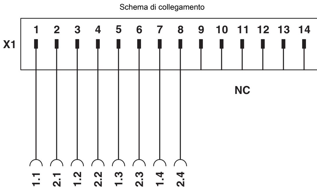
Schema di collegamento FLKM 14-PA-INLINE/DIO8
