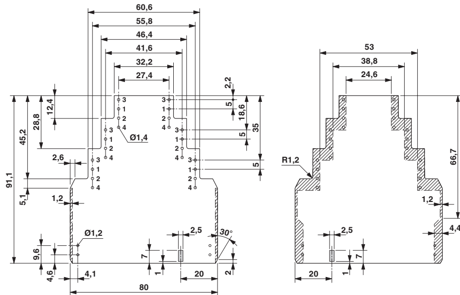
Disegno quotato
