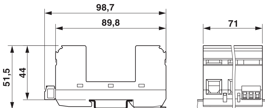
Disegno quotato
