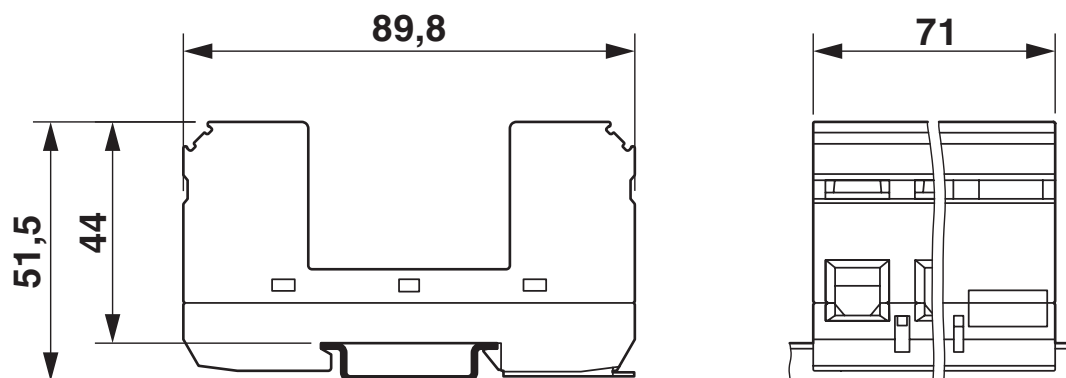
Disegno quotato
