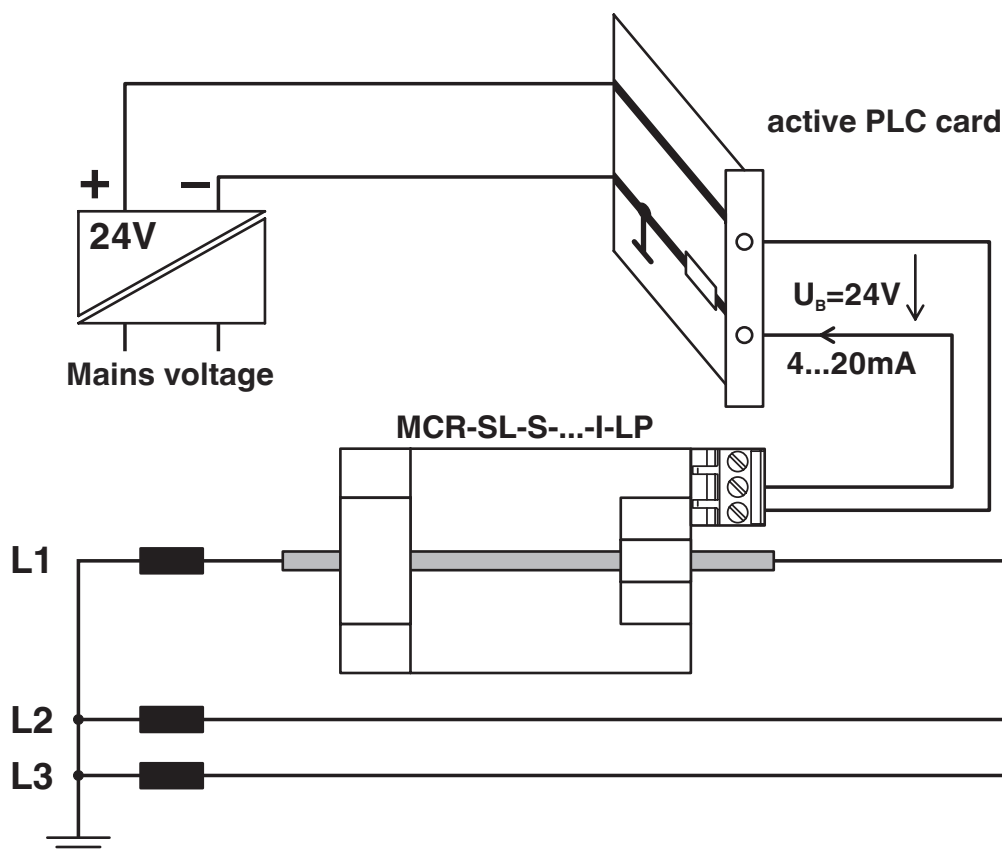
Disegno applicazione
