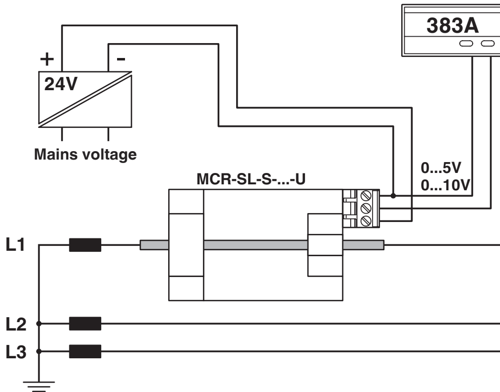
Disegno applicazione
