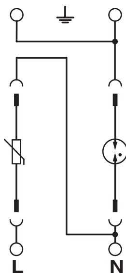
Schema di collegamento
