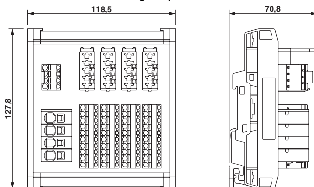
Disegno quotato
