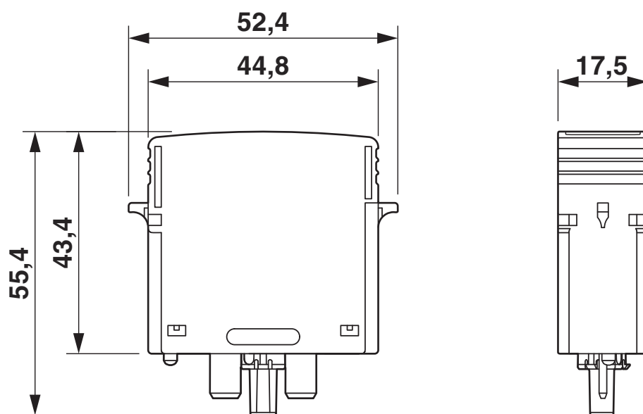
Disegno quotato
