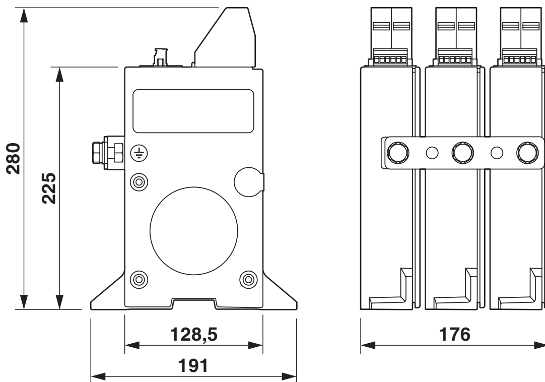
Disegno quotato
