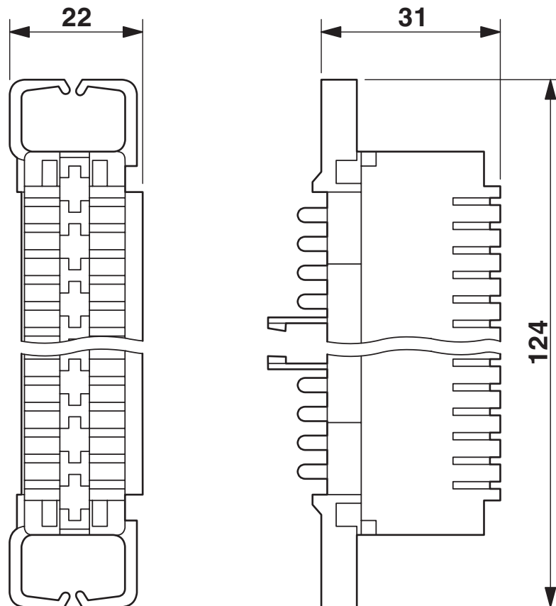
Disegno quotato
