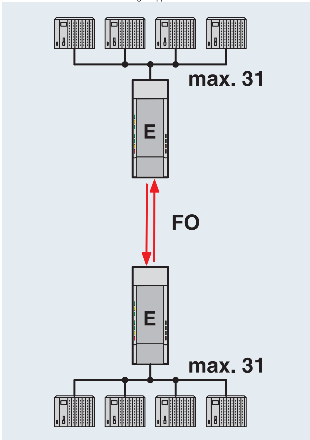
Collegamento punto-punto
