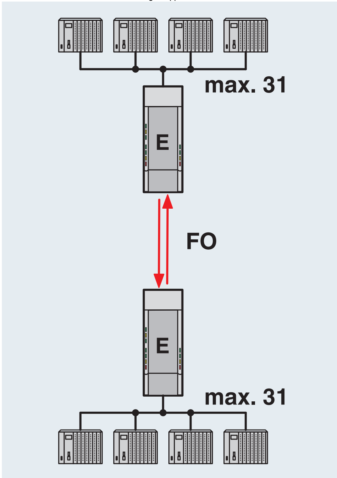
Collegamento punto-punto
