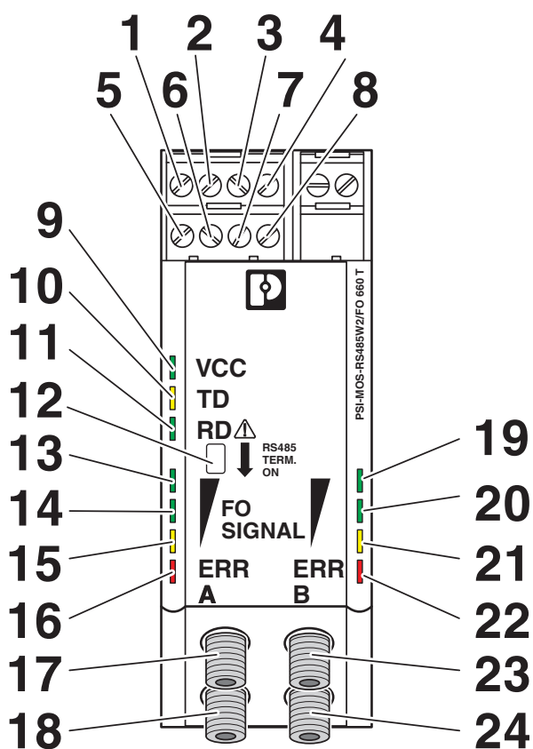
Disegno schema
