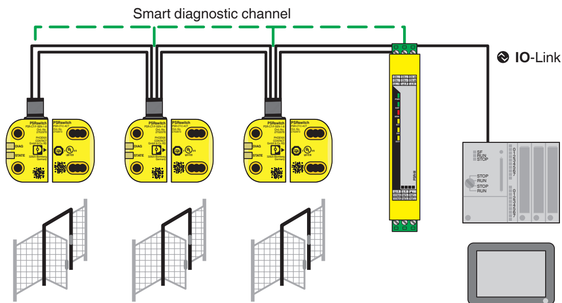
Disegno applicazione
