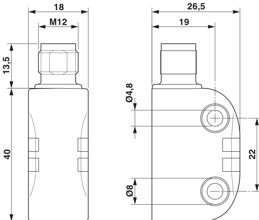
Disegno quotato
