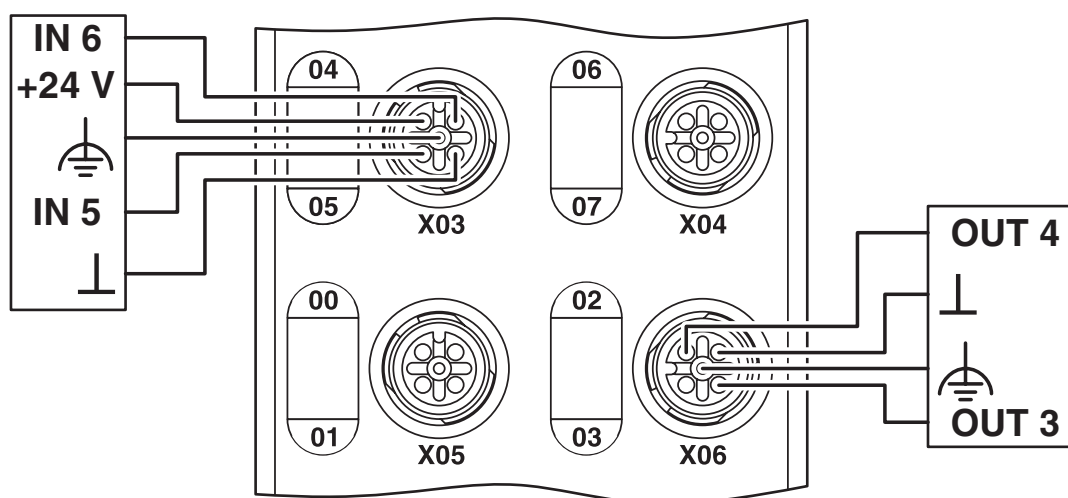
Disegno collegamento
