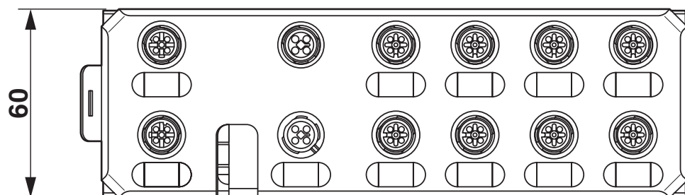
Disegno collegamento
