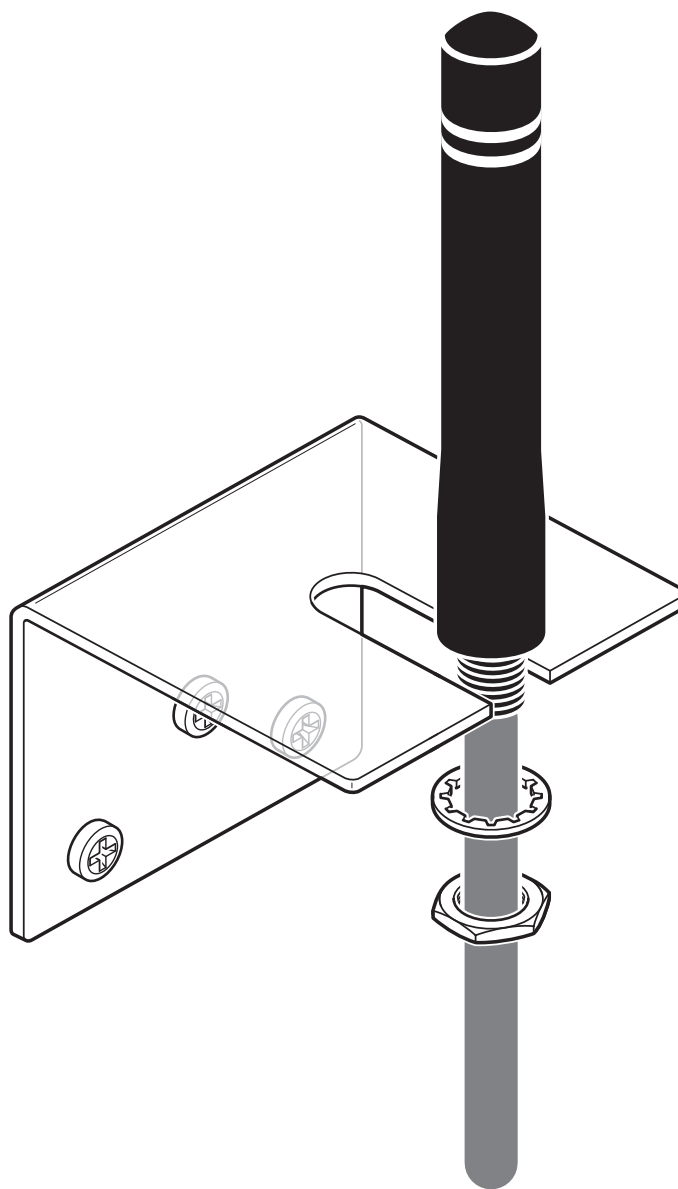
Disegno schema
