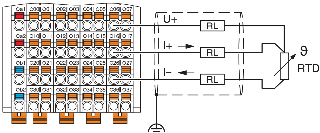
Disegno collegamento
