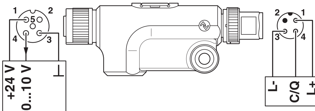
Disegno collegamento
