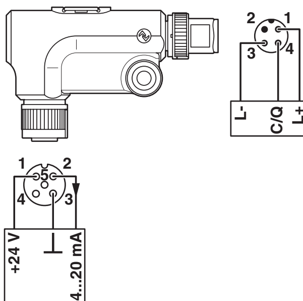
Disegno collegamento
