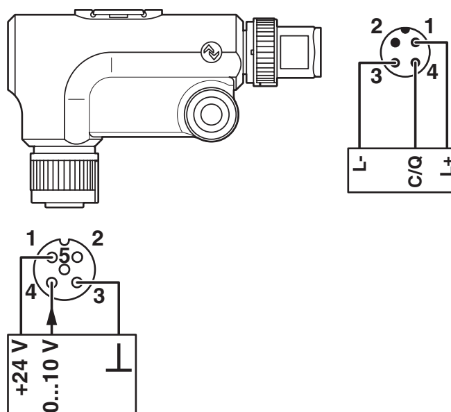
Disegno collegamento
