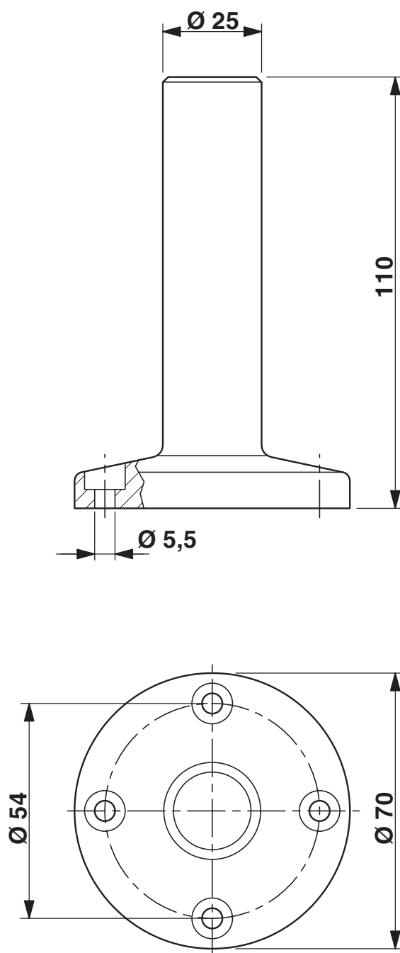
Disegno quotato
