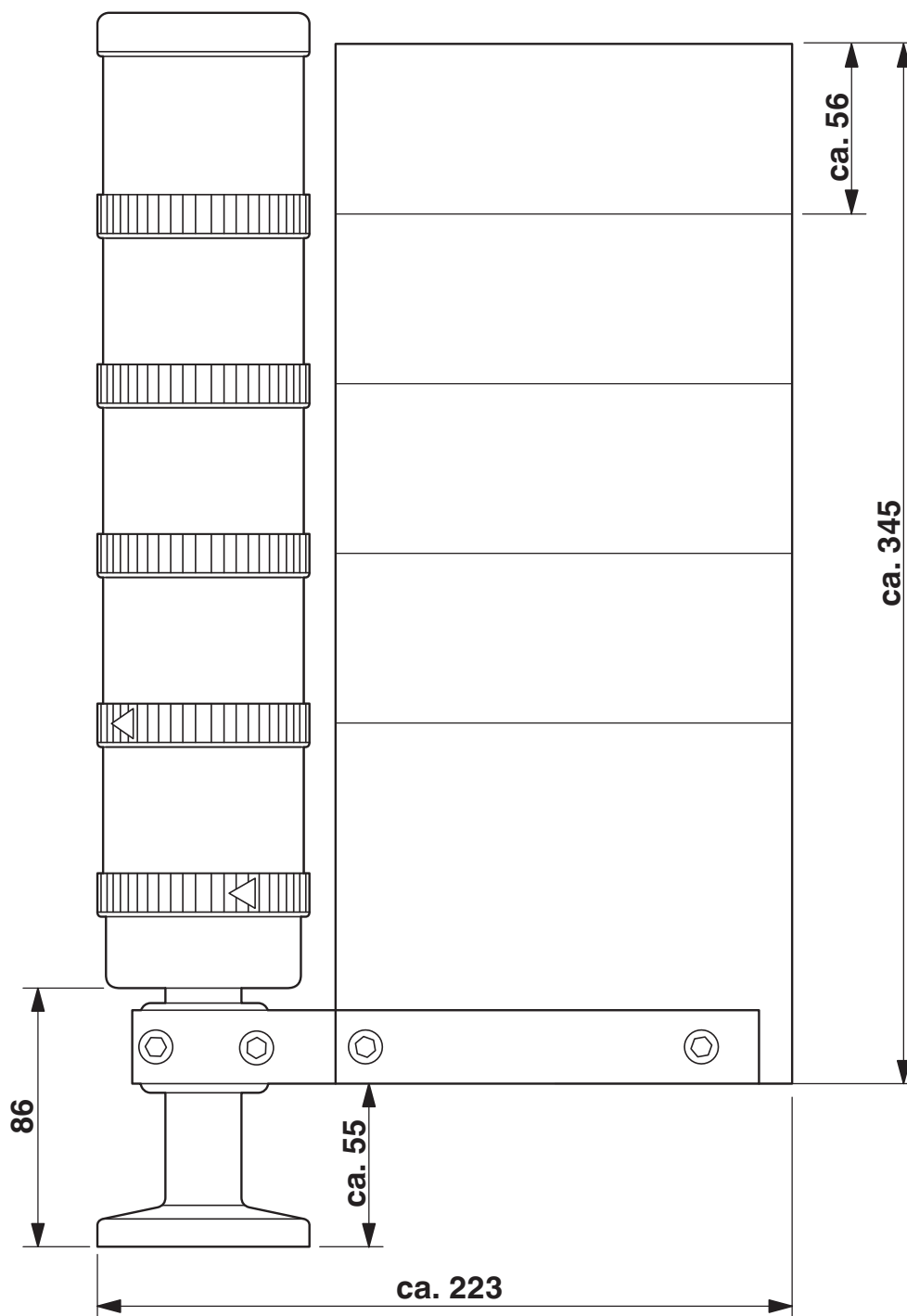
Disegno quotato
