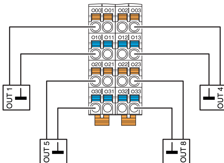
Disegno collegamento
