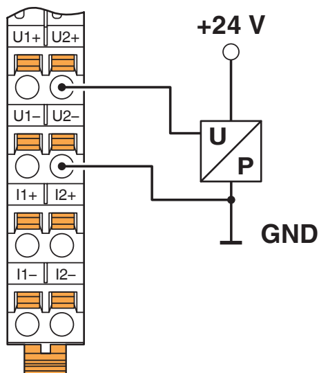
Disegno collegamento
