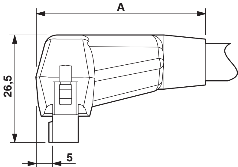
Disegno quotato
