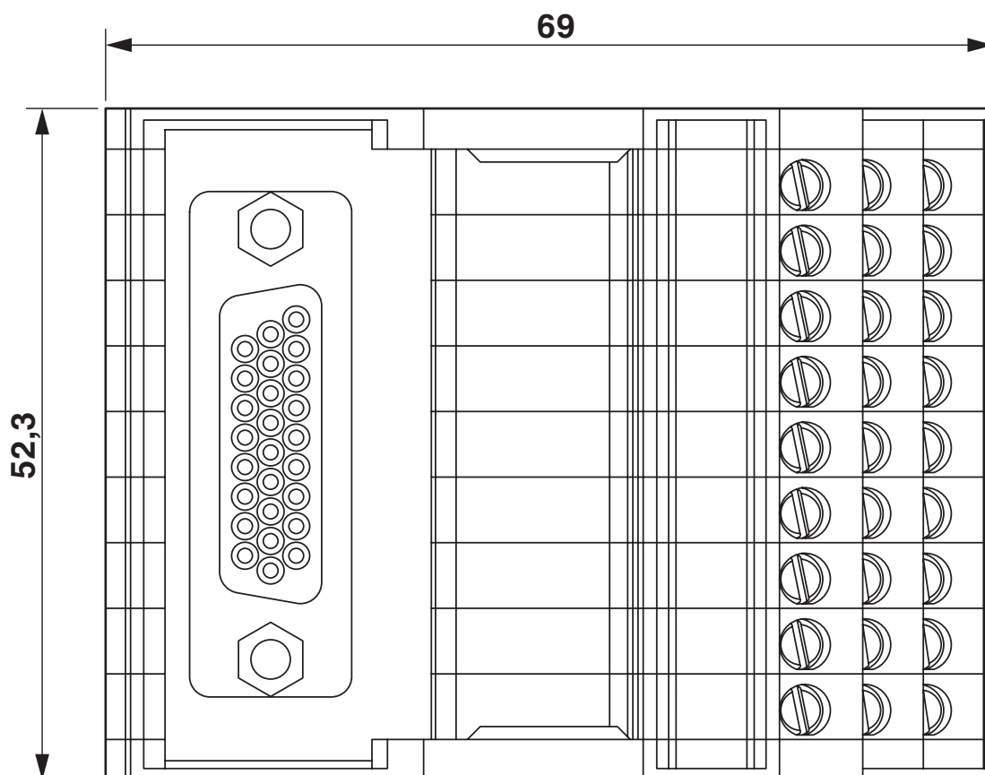
Disegno quotato
