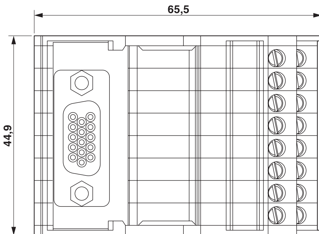
Disegno quotato
