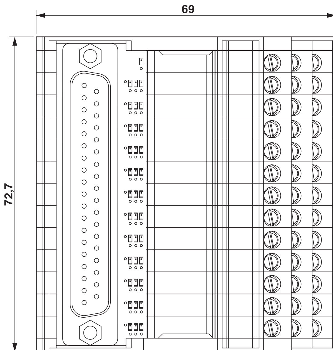
Disegno quotato
