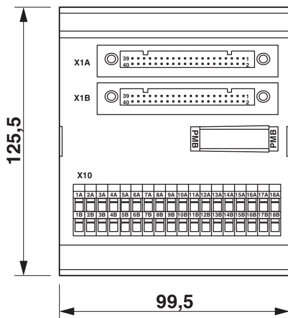
Disegno quotato
