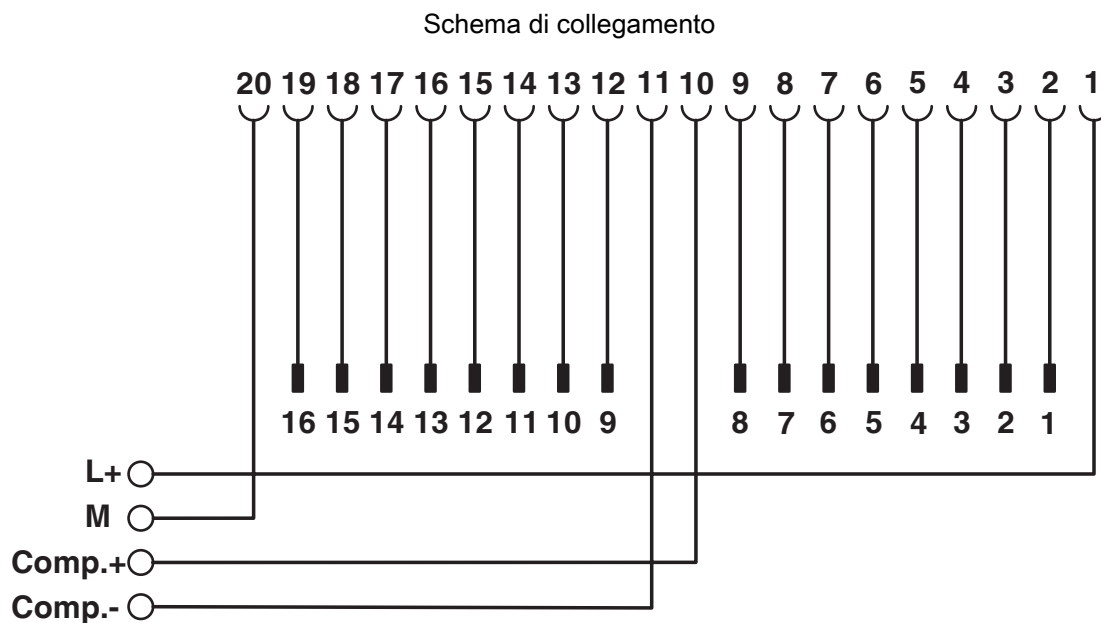
Schema di collegamento FLKM 16-PA-S300/MINI-MCR
