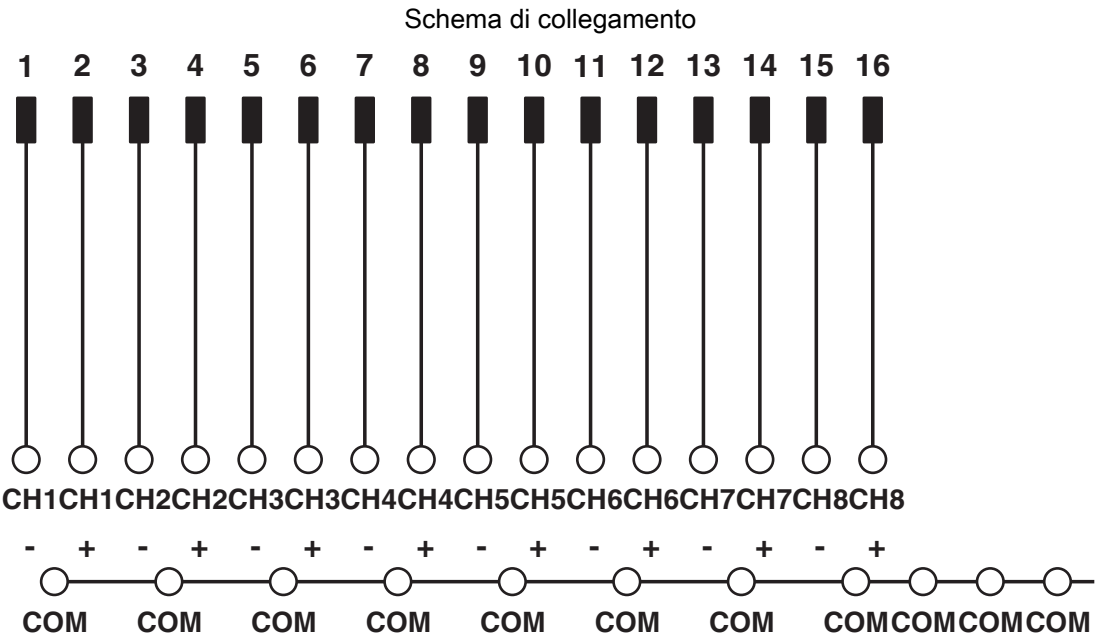
Schema di collegamento FLKM 16/AI/DV
