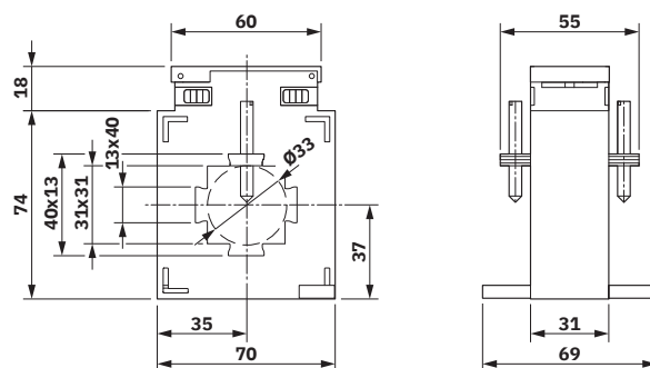
Disegno quotato
