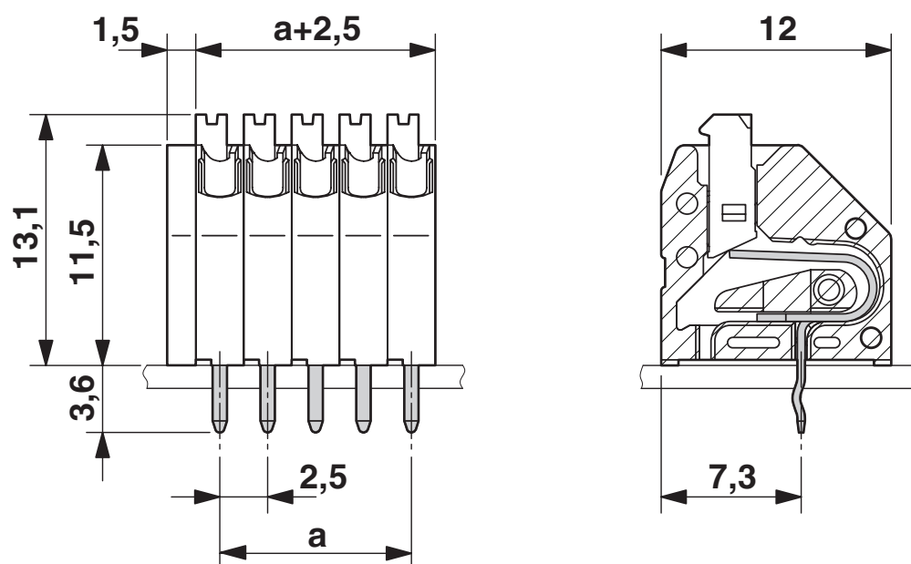
Disegno quotato
