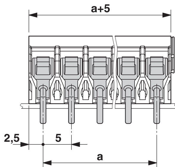
Disegno quotato
