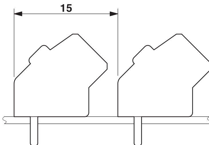
Disegno quotato
