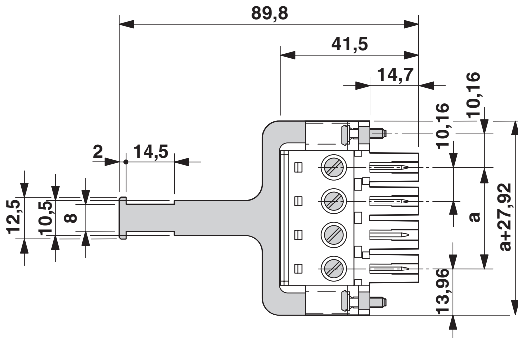
Disegno quotato
