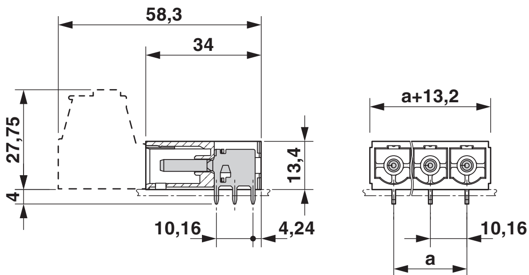
Disegno quotato
