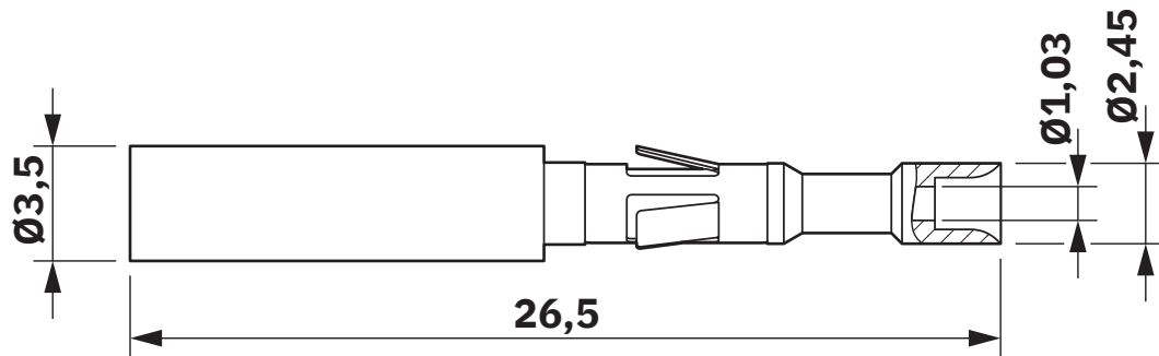
Disegno quotato
