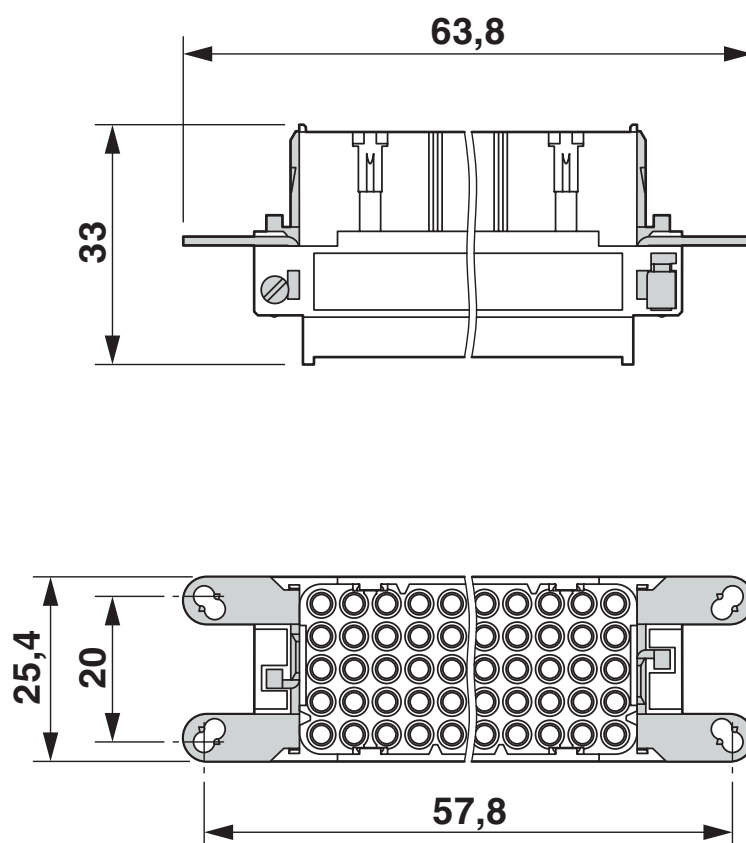
Disegno quotato
