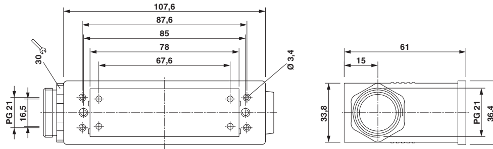
Disegno quotato
