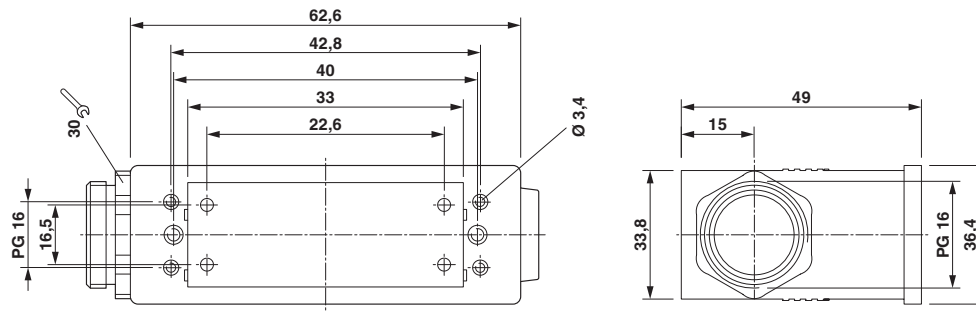
Disegno quotato
