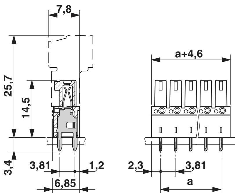
Disegno quotato
