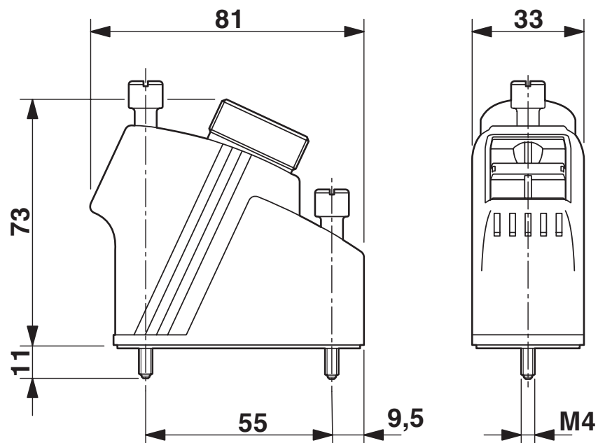
Disegno quotato
