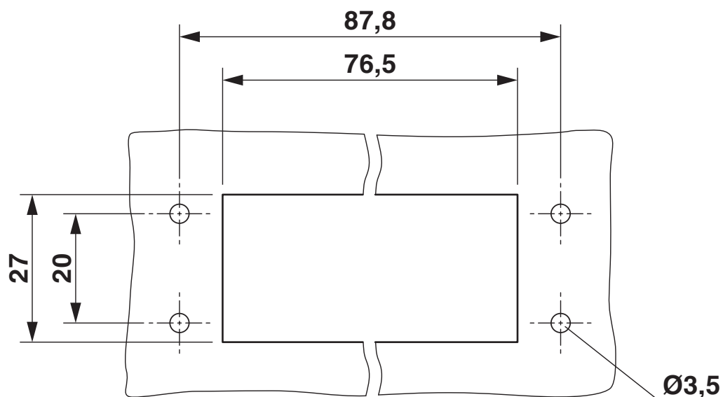
Disegno quotato
