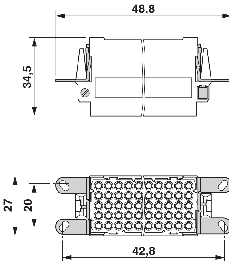
Disegno quotato
