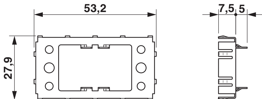
Disegno quotato
