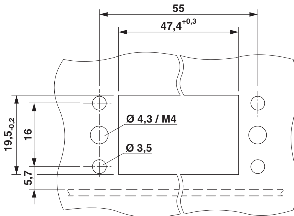
Disegno quotato
